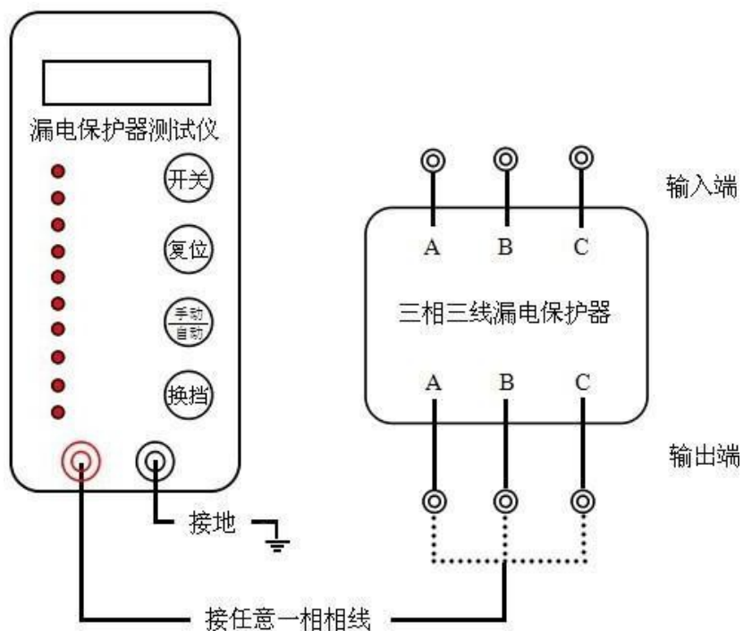
图 2 三相三线接线法
