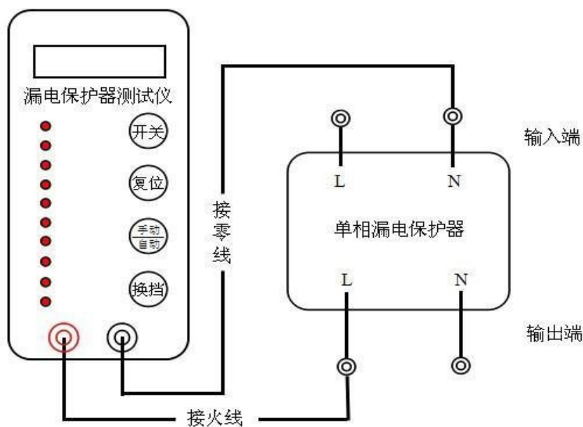
图 1 单相接线法
